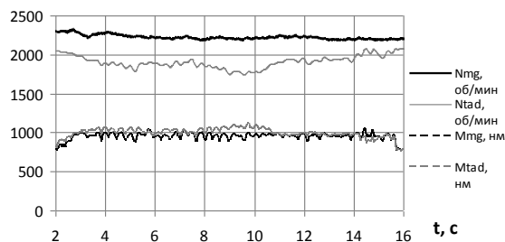
Рис. 1. Временные диаграммы работы трактора «БЕЛАРУС–3023» в режиме пахоты с максимальной мощностью
